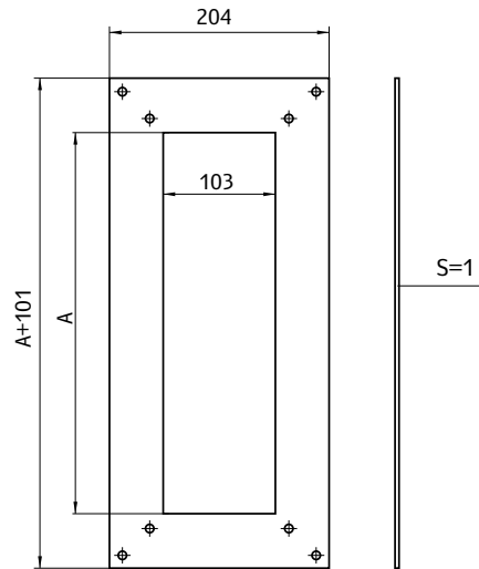
Пластина - переход
